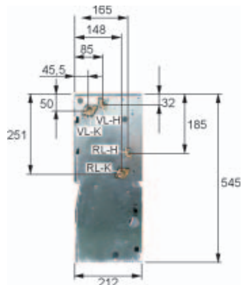
4-Leiter-System 3 RR Kühlen / 1 RR Heizen
